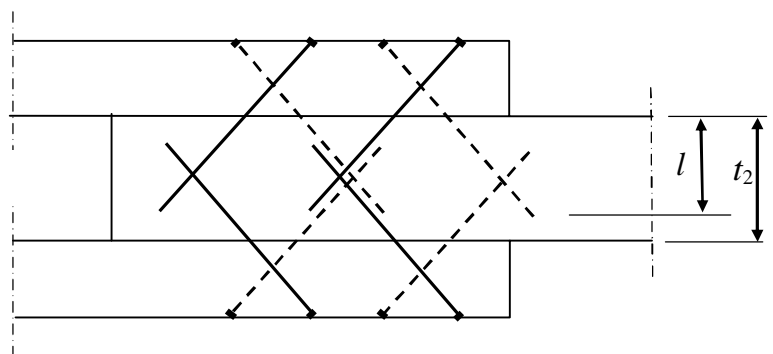
Kuva C.4 Limittyvät ruuvit.
