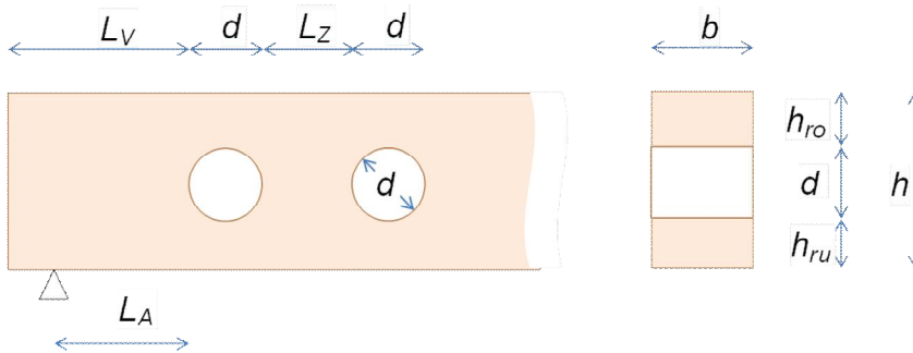
Kuva A1. Pyöreään reikään liittyvät merkinnät.
