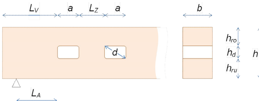
Kuva A2. Suorakaiteen muotoiseen reikään liittyvät merkinnät.
