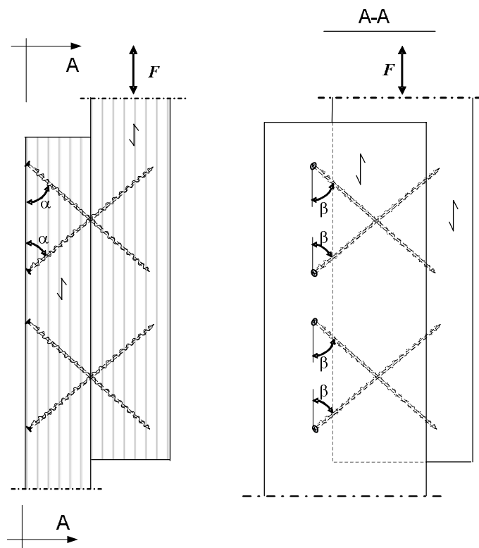
Kuva C.3. Kolmiulotteinen vinoruuviliitos.
