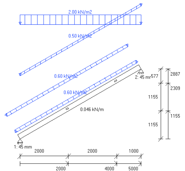
Kerto-Ripa® -kattorakenne
